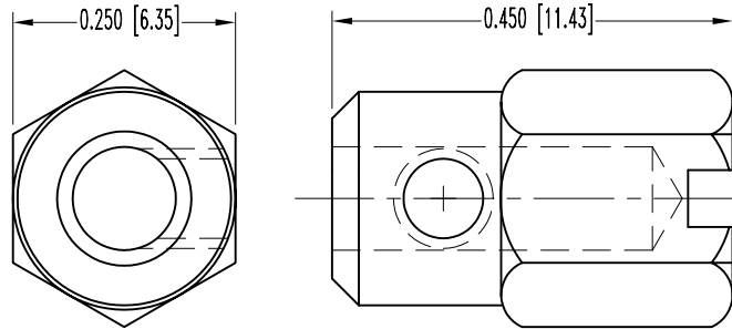
2X HEX KNOB
