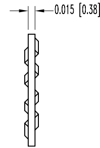
LOCKWASHER
